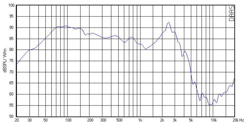
Frequenzgang XAW 310 HC
